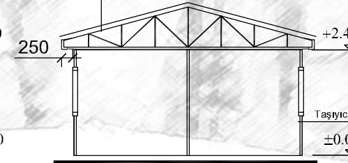
A-A KESİTİ
