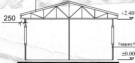
A-A KESİTİ
