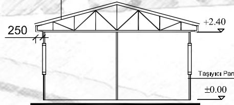
A-A KESİTİ
