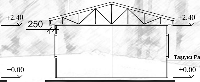
A-A KESİTİ
