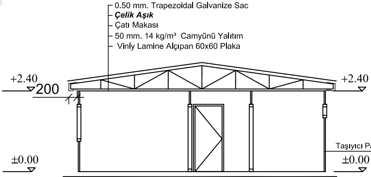
A-A KESİTİ
