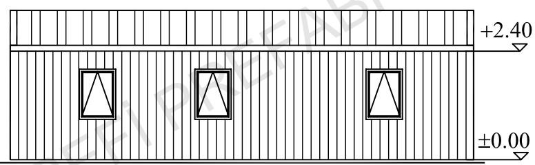
CEPHE GÖRÜNÜŞÜ
