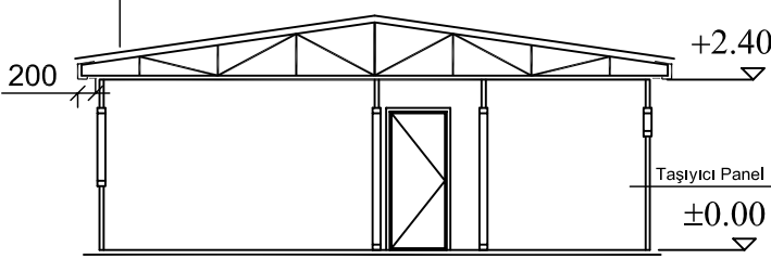
A-A KESİTİ
